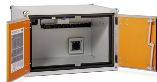
Produkt Frontalansicht offen mit beispielhaftem Inhalt bzw. mit Zubehör (nicht im Lieferumfang enthalten)
